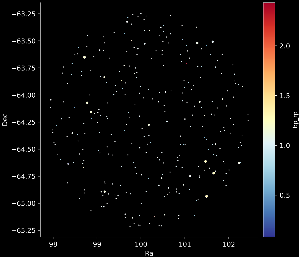
GALAH DR4 Field: [6966] Stars: 305
